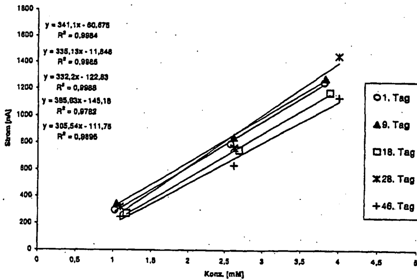
Abbildung 14: Sensitivität von TMPD-modifizierten Glukosebiosensoren mit PVP-Schutzschicht in Abhängigkeit des Sensoralters
